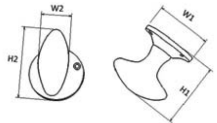
Raglan Door Knob
